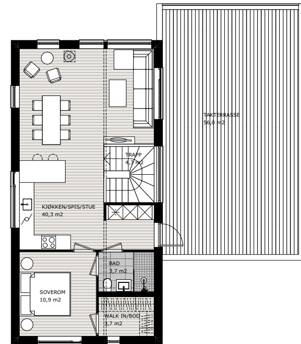
2. ETASJE
